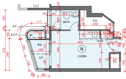
8-9/F Part Plan of Flat N 8-9樓N單位部分平面圖
