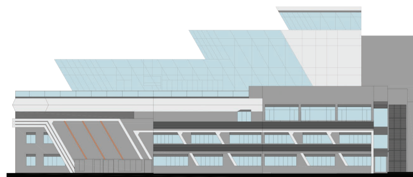
Elevation Plan 6- Podium 立面圖6 - 平台
