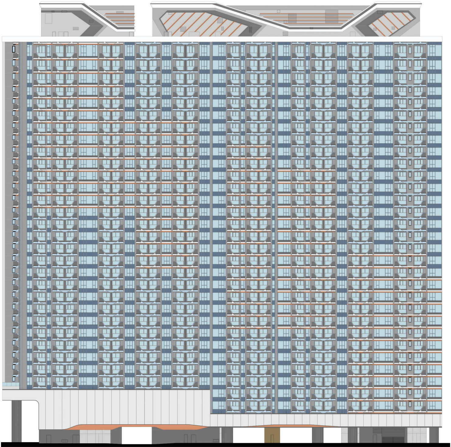
Elevation Plan 1 - Tower 1 (Tower 1A, Tower 1B, Tower 1C) 立面圖1 - 第1座(第1A座、第1B座、第1C座)
