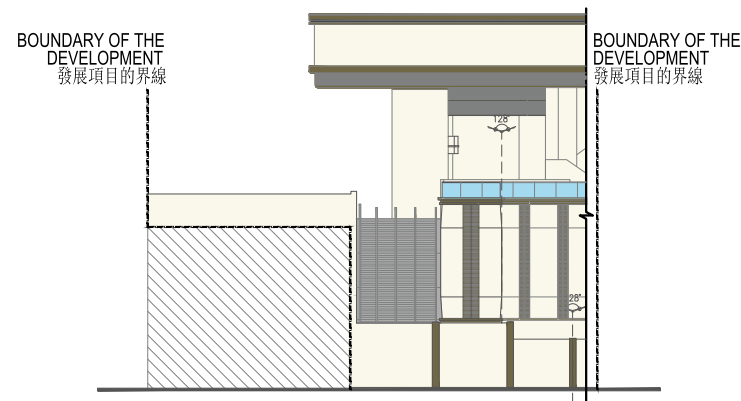
Elevation E4 立面圖 E4
