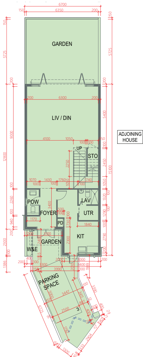
GROUND FLOOR 地下
