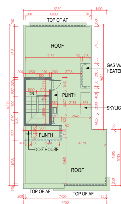
ROOF 天台
