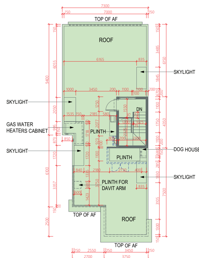
ROOF 天台
