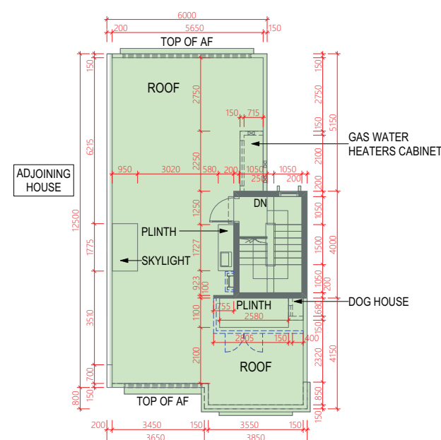
ROOF 天台
