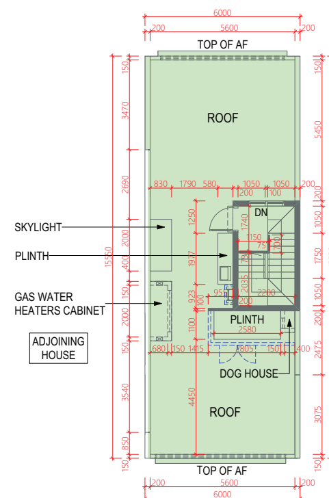
ROOF 天台
