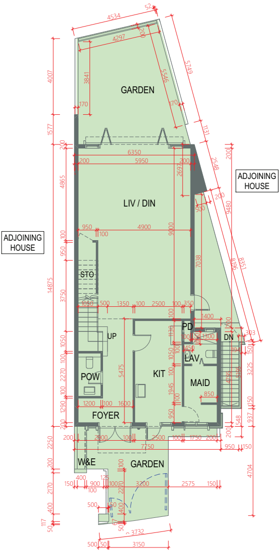
GROUND FLOOR 地下
