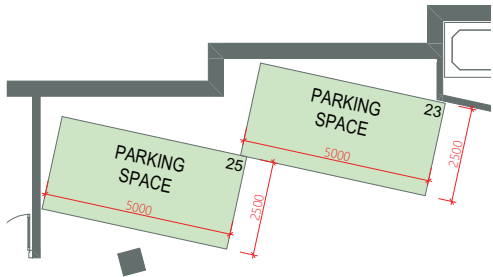
PART PLAN OF CARPARK FLOOR 停車場層部份平面圖
