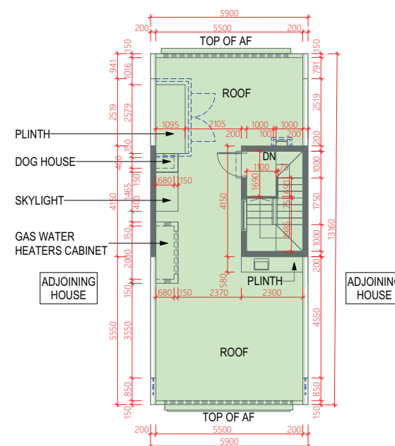
ROOF 天台
