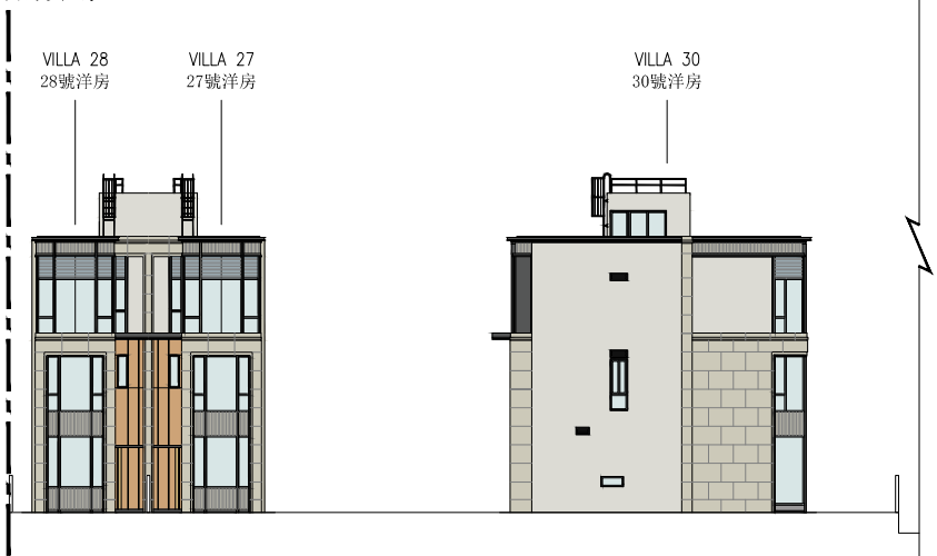
Elevation Plan C 立面圖 C
