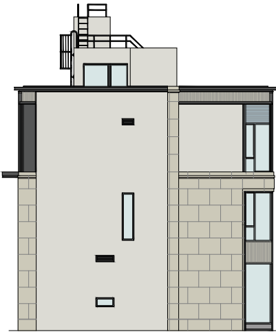
Elevation Plan C 立面圖 C (For Villa 26 Only) (只適用於26號洋房)
